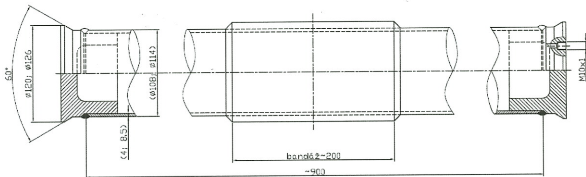
Obr. 1: Původní vzorek ze zkoušek v roce 2018
