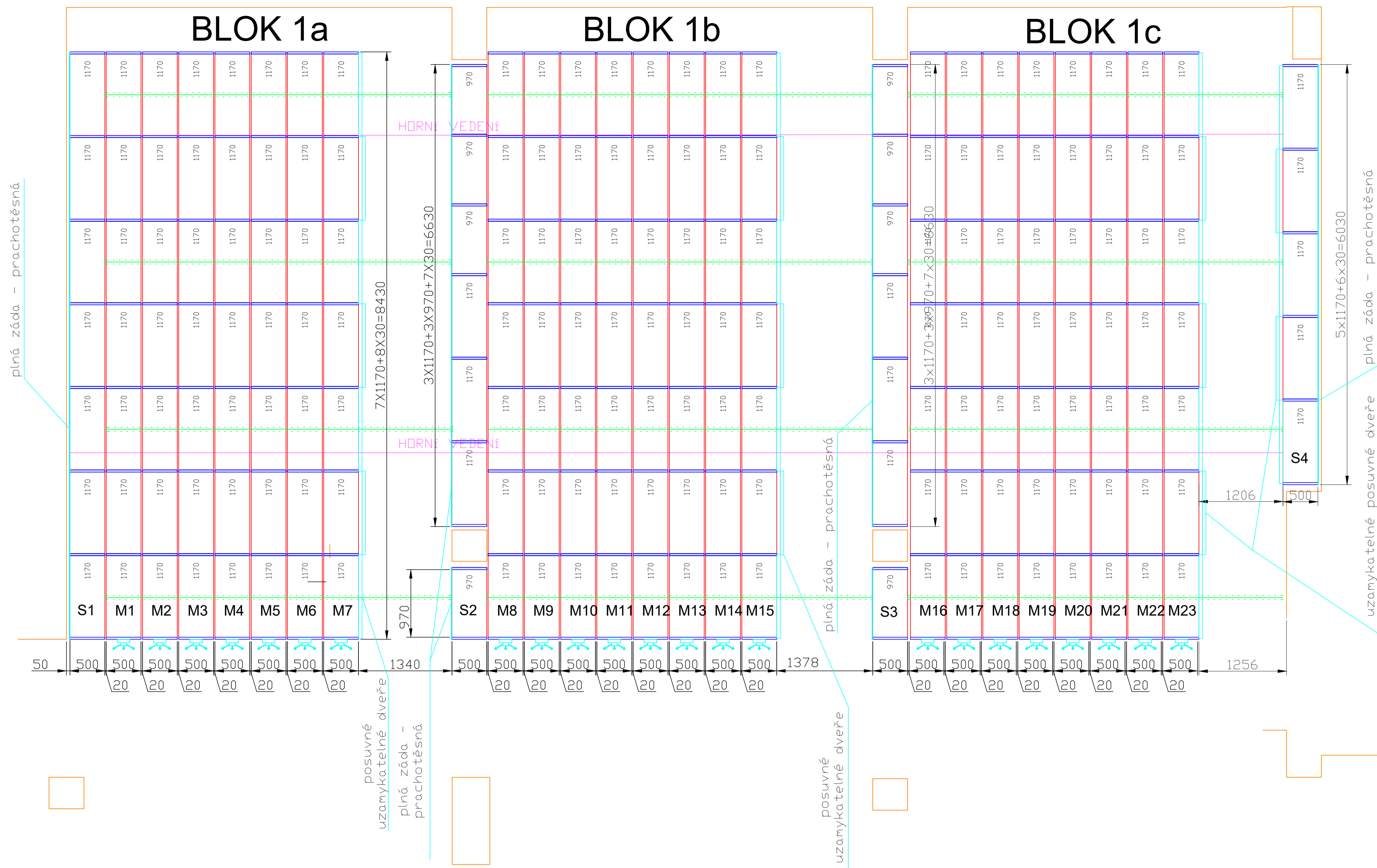
VÝŠKOVÉ ČLENĚNÍ BLOK 1b Mobilní regály 1170x5002R - 155KG 970x5001R - 180KG
