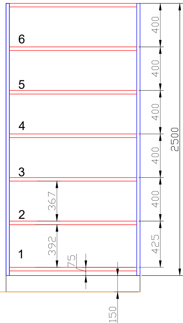
VÝŠKOVÉ ČLENĚNÍ BLOK 1b Stacionární regály 1170x5002R - 155KG 970x5001R - 180KG
