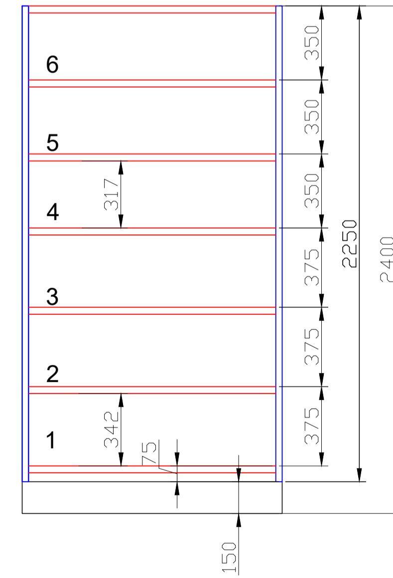
VÝŠKOVÉ ČLENĚNÍ BLOK 1a,1c Stacionární regály 1170x5002R - 155KG 970x5001R - 180KG
