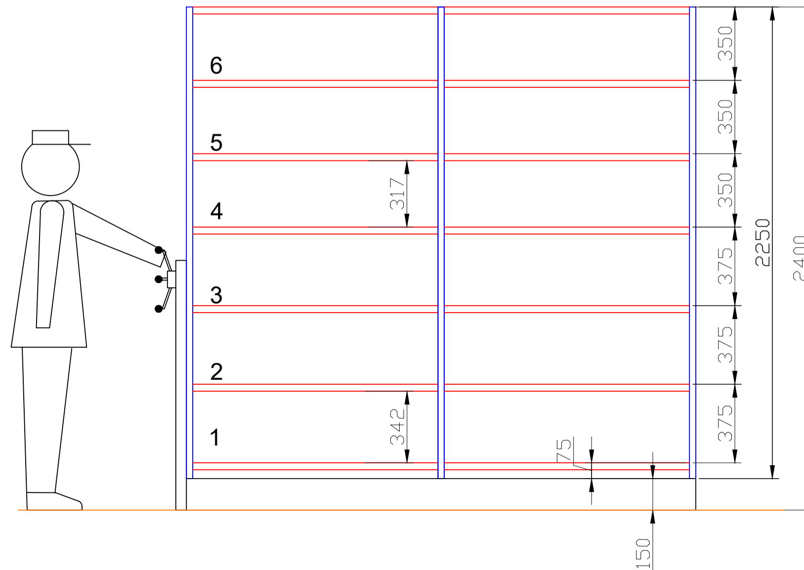
VÝŠKOVÉ ČLENĚNÍ BLOK 1a,1c Mobilní regály 1170x5002R - 155KG 970x5001R - 180KG
