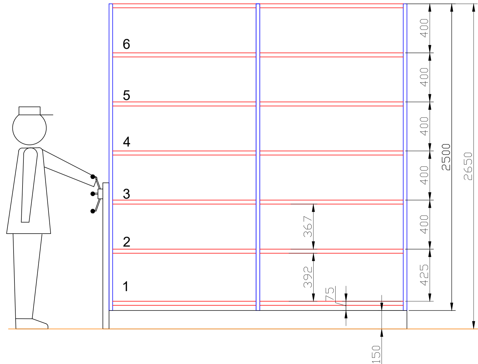
VÝŠKOVÉ ČLENĚNÍ BLOK 1b Mobilní regály 1170x5002R - 155KG 970x5001R - 180KG
