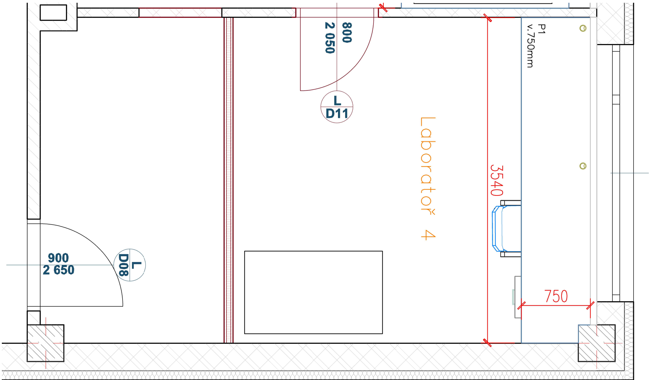
Laboratoř 4 – pŮdorys
